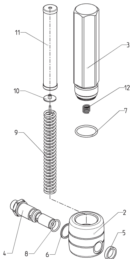
Reservebillede, højtryksfilter
