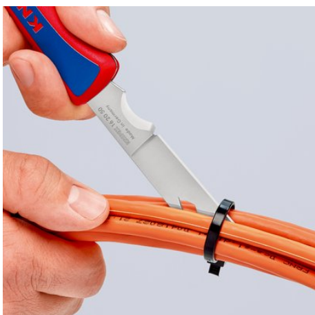
Elektrikerfoldekniven er altid lige ved hånden og velegnet til alle gængske skæreopgaver
