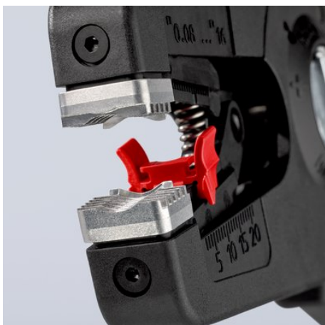
Halvrunde holdekæber med kamprofil sikrer bedre greb og holder alle isoleringsmaterialer sikkert fast
