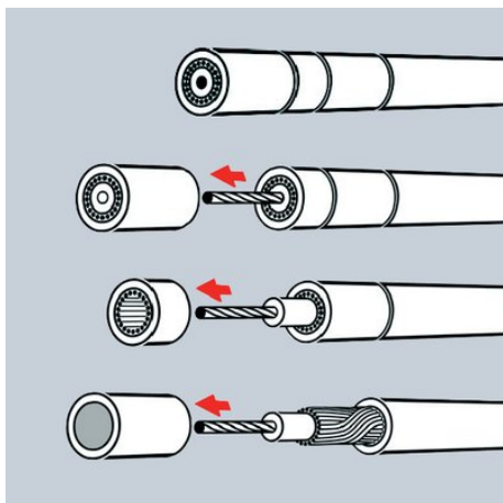
Tretrinnet afisolering af koaksial-kabel
