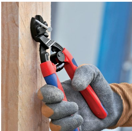
20° bøjet hoved med ensidig lask og sidesnit til plan afskæring, med fri plads til at gribe fat
