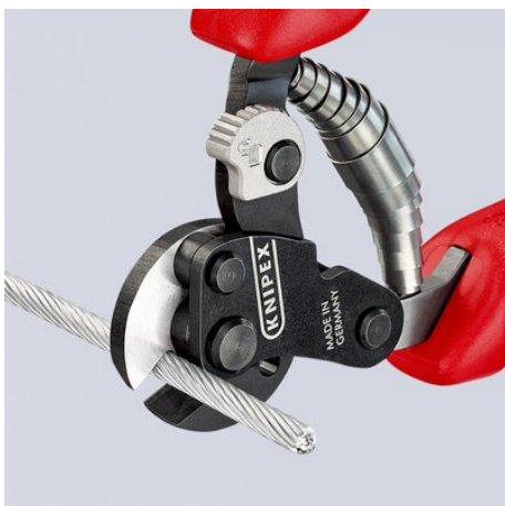
Skæring af ekstra faste stålwirer (1960 N/mm 2 ) op til 4 mm Ø
