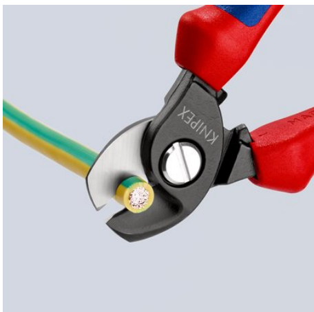
Kabelsnit med kabelsaks: let, pænt og ordentligt snit uden at deformere kablet
